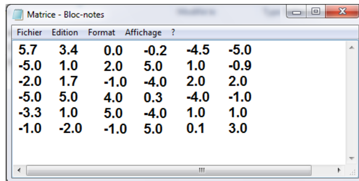
Matrice carrée inversible d'ordre 6, stockée dans un fichier texte
